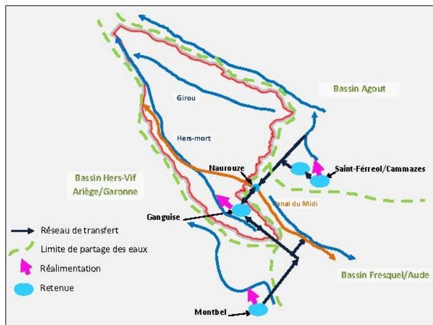
Figure II. 2 : Schéma des transferts interbassins autour de la retenue de la Ganguise
